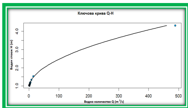
Фигура 1. Ключова крива Q-H (метод bdrс).
