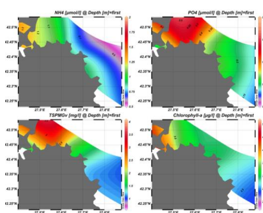
Фигура 2. Градиент на еутрофикация по южното крайбрежие на Бургаския залив (2009–2024 г.).
